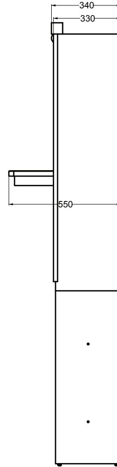
VISTA LATERALE
