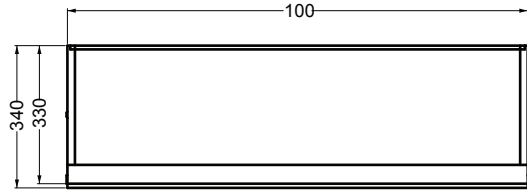
PIANTA
