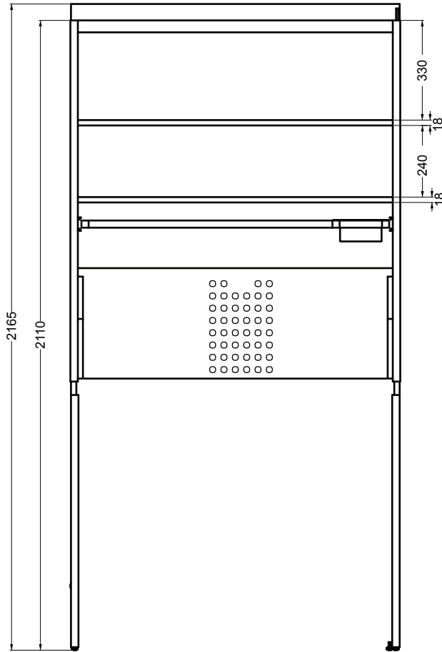
VISTA FRONTALE
