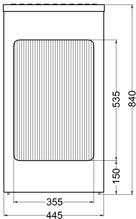
VISTA FRONTALE
