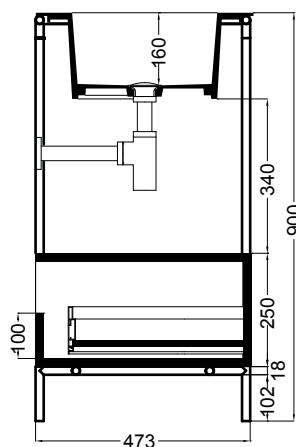
SEZIONE A-A'
