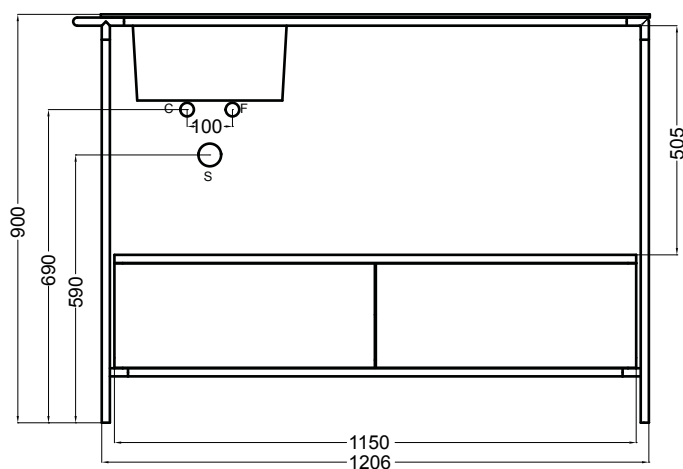
VISTA FRONTALE
